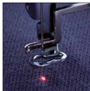
Вышивальная лапка с LED указкой
